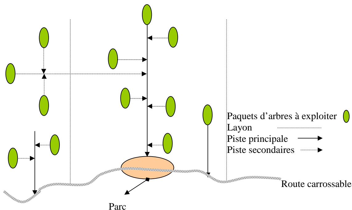
Figure 3 : Planification du réseau des pistes de débardage
