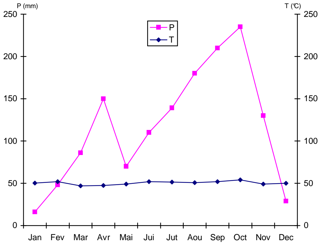
Fig 1 : Diagramme Ombrothermique de Yokadouma
